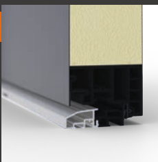
Próg aluminiowy z przekładką termiczną
